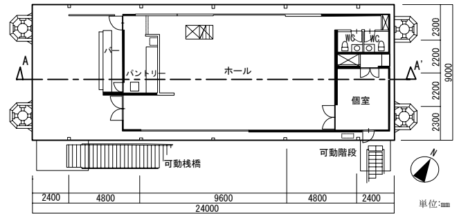
図-2 「レストラン船」(当事例)平面図
