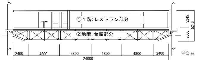
図-3 「レストラン船」(当事例)A-A' 断面図
